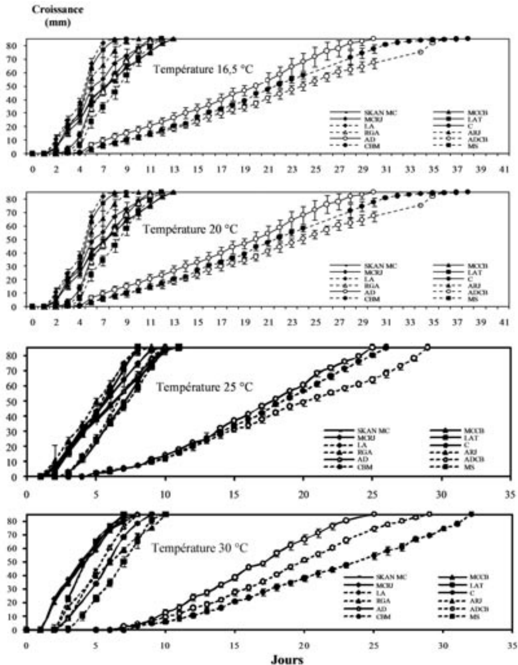
Fig. 1. Evolution de la croissance mycélienne de Meristacrum (MCRJ, SKANMC, MCCB), d' Arthrotritys oligospora (LAT, LA), d' A. conoides (C, RGA), d' A. musiformis (ARJ), d' A. dactyloides (AD, ADCB), de Monacrosporium rutgeriensis (MS) et de M. cionopagum (CBM) aux températures de 16,5, 20, 25, 30°C. Les barres correspondent aux intervalles de confiance à P = 0,05.
