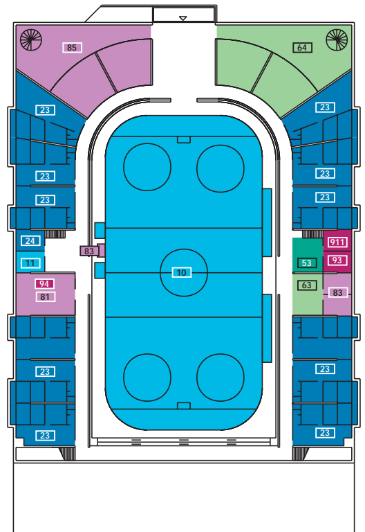
rez de chaussée - niveau glace (1:1000)
