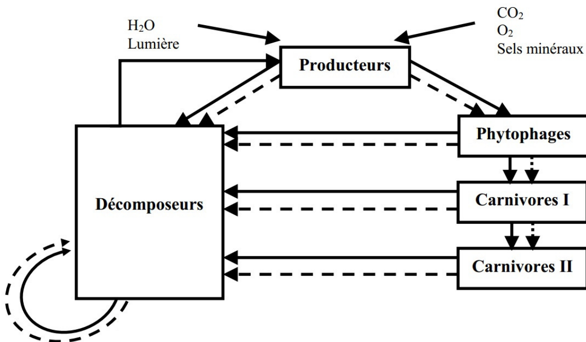
Figure (03): Schéma de la structure globale d'une chaîne alimentaire. Circulation de la matière (trait continu) et de l'énergie (trait discontinu).
