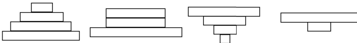
Figure (02): Diverse schématisation des pyramides écologiques.
